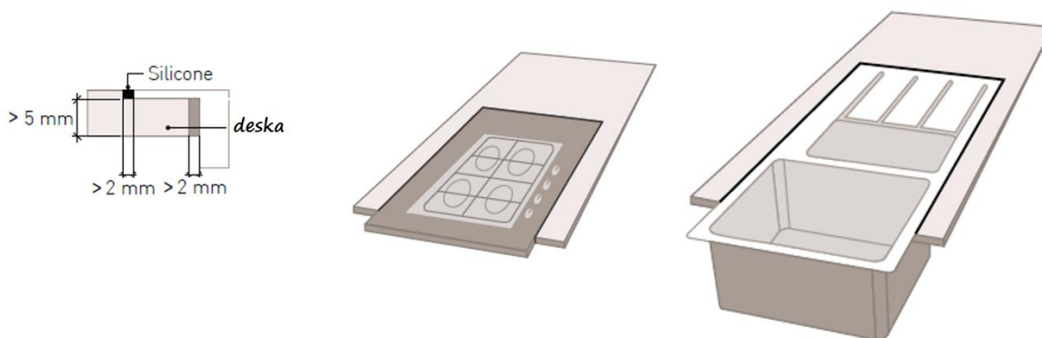
Obrázek č. 2 – usazení prvků do roviny
