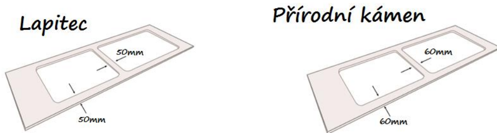
Obrázek č. 5 – minimální vzdálenost okraje od výřezů
